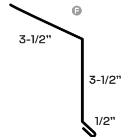
405 Drip Edge Specify Pitch
