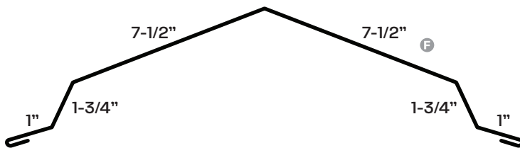
491 Ridge Cap Specify Pitch
