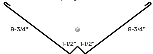
402 Valley Specify Pitch
