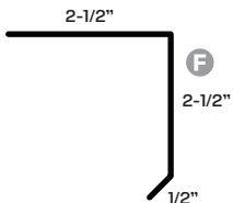
109 Drip Edge
