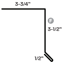
105 Drip Edge
