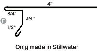
129 NE Drip Edge
