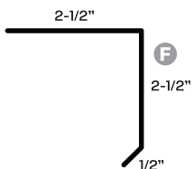
109 Drip Edge
